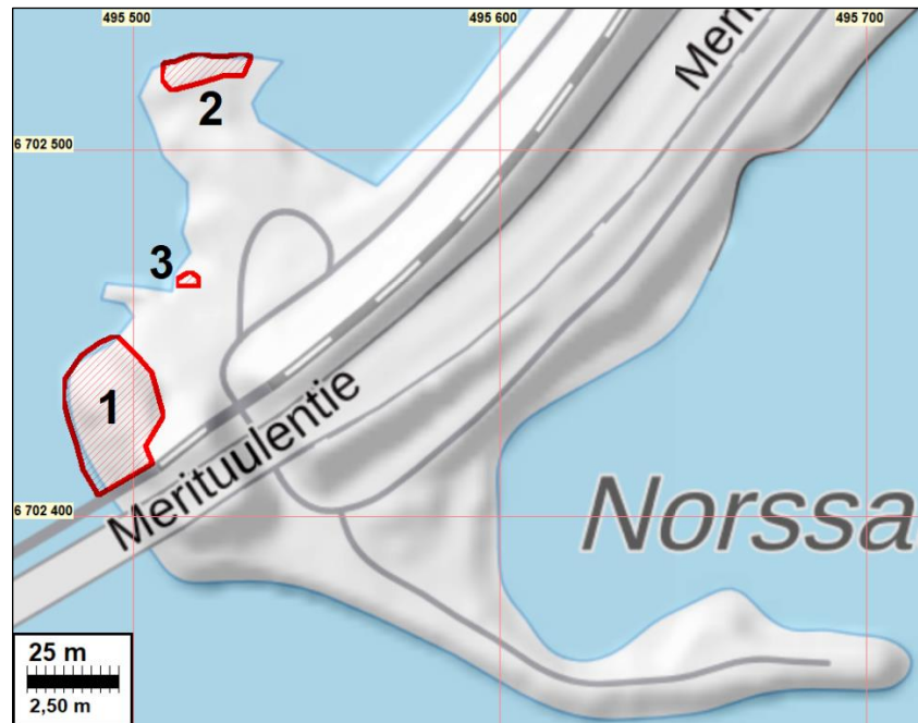
Norssaaren kalliohakkauskohteet 1-3
